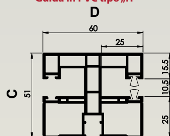
Guida in PVC tipo „H“
